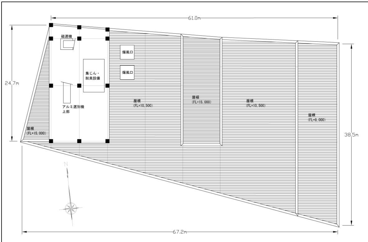
図 4 - 5 配置計画案 ( 4 F )
